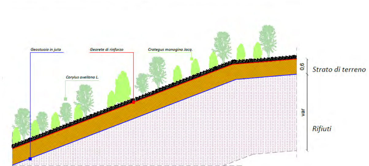
Particolare copertura evapotraspirativa corpo discarica : copertura sulle scarpate - scala 1:50
